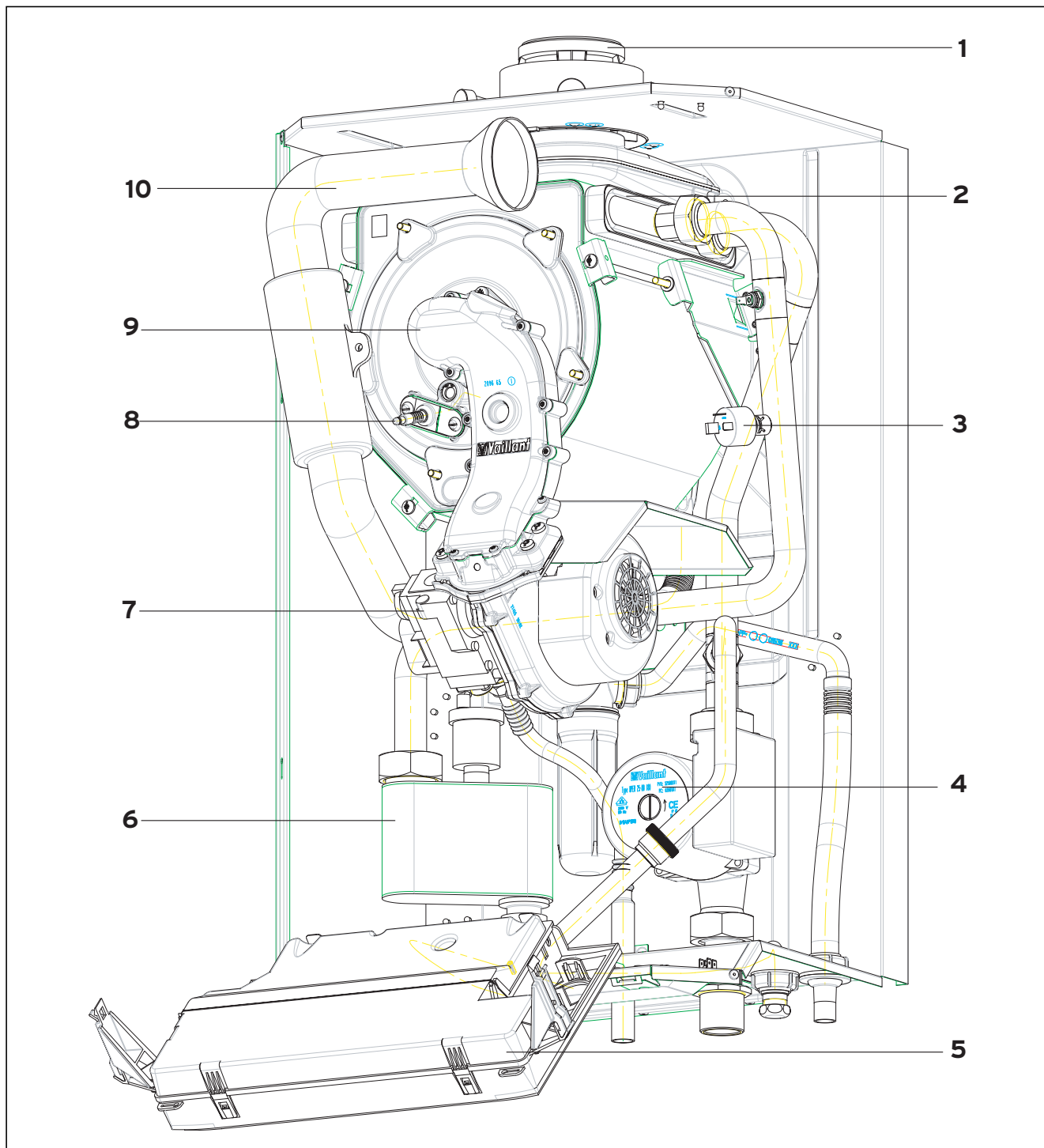
Рис. 1.1 Функциональные элементы
