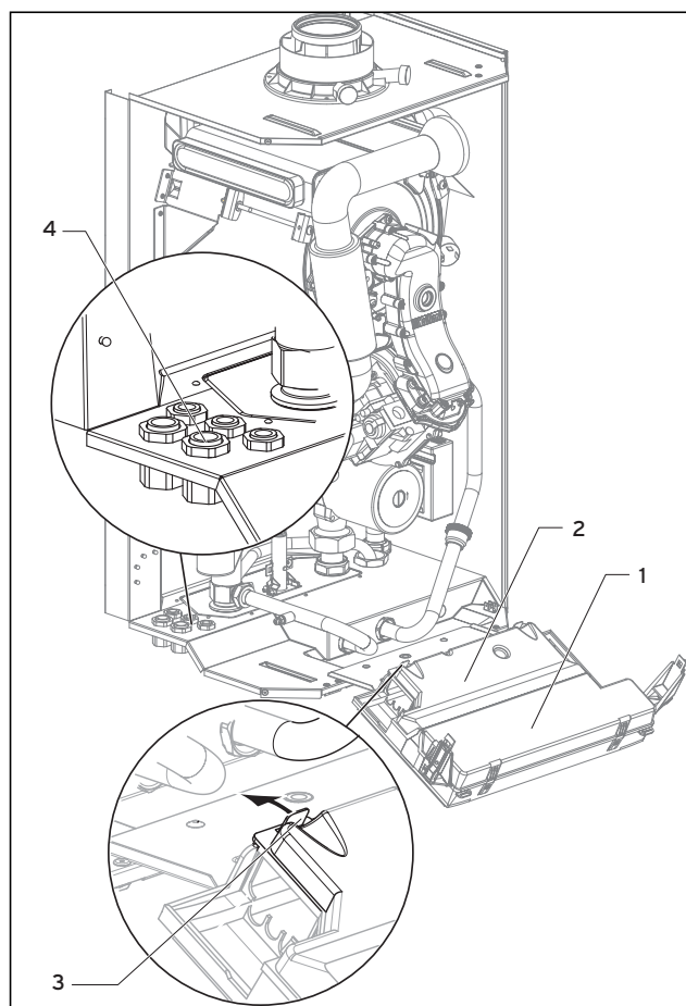
Рис. 4.9 Открывание задней крышки электронного блока
