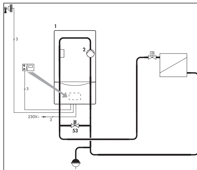
Рис. 4.1 Пример 1: Радиаторное отопление; прямое подключение насос внутри аппарата
