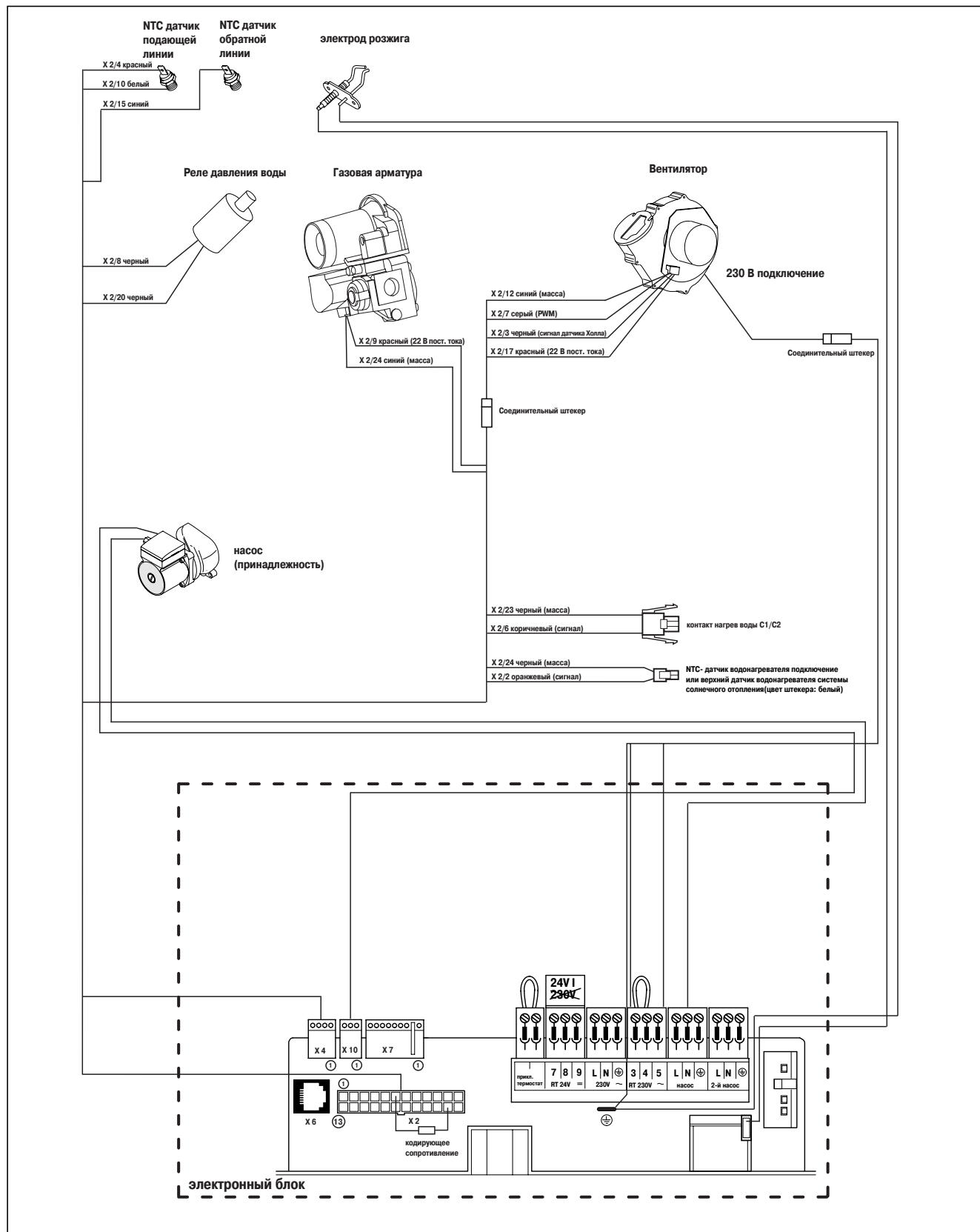
Рис. 4.12 Монтажная схема аппарата esotec VU 466
