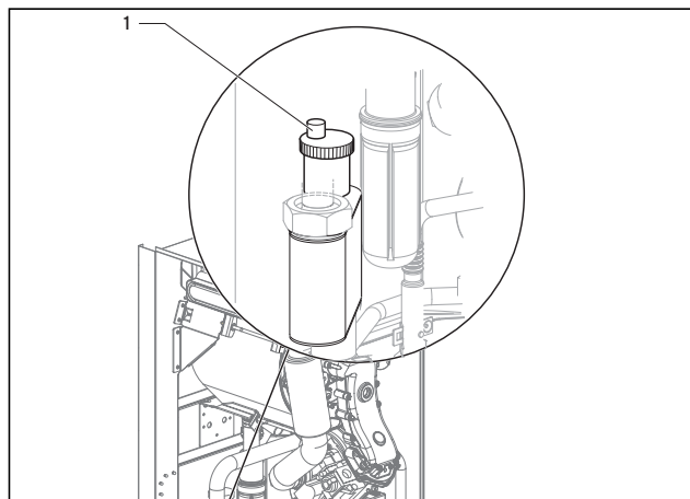
Рис. 5.1 Удаление воздуха из аппарата
