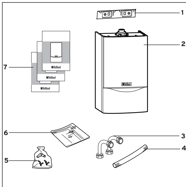
Рис. 3.1. Комплект поставки
