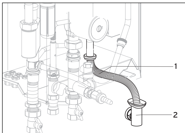
Рис. 4.9 Отвод конденсата
