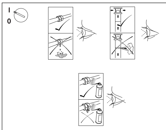
Рис. 5.5 Проверка функционирования
