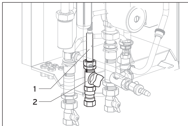
Рис. 4.6 Подключение газа (возможен только открытый монтаж)
