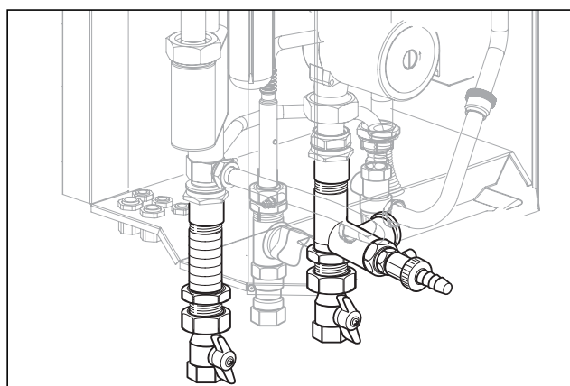
Рис. 4.7 Подключение подающей и обратной линии системы отопления
